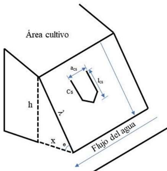
Figura 1. Bosquejo de un drenaje terciario. y: profundidad del drenaje. x: distancia horizontal en relación a la altura. h: talud del drenaje. c: cajuela delimitación y recolección de sedimentos. L: longitud de la pendiente.
