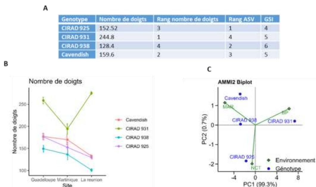
Figure 1. Nombre de doigts A. Valeurs d'ASV et GSI par genotype B. Normes de réaction C. Biplot du modèle AMMI
