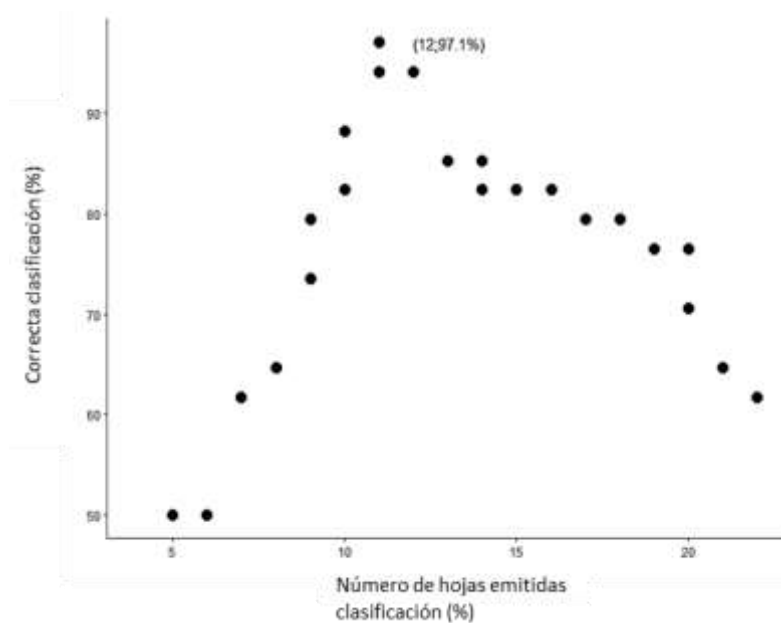
Figura 5. Progreso de la correcta clasificación (97.1%), utilizando el punto de corte obtenido como separador entre la fase vegetativa y reproductiva, en la emisión de la hoja # 12.
